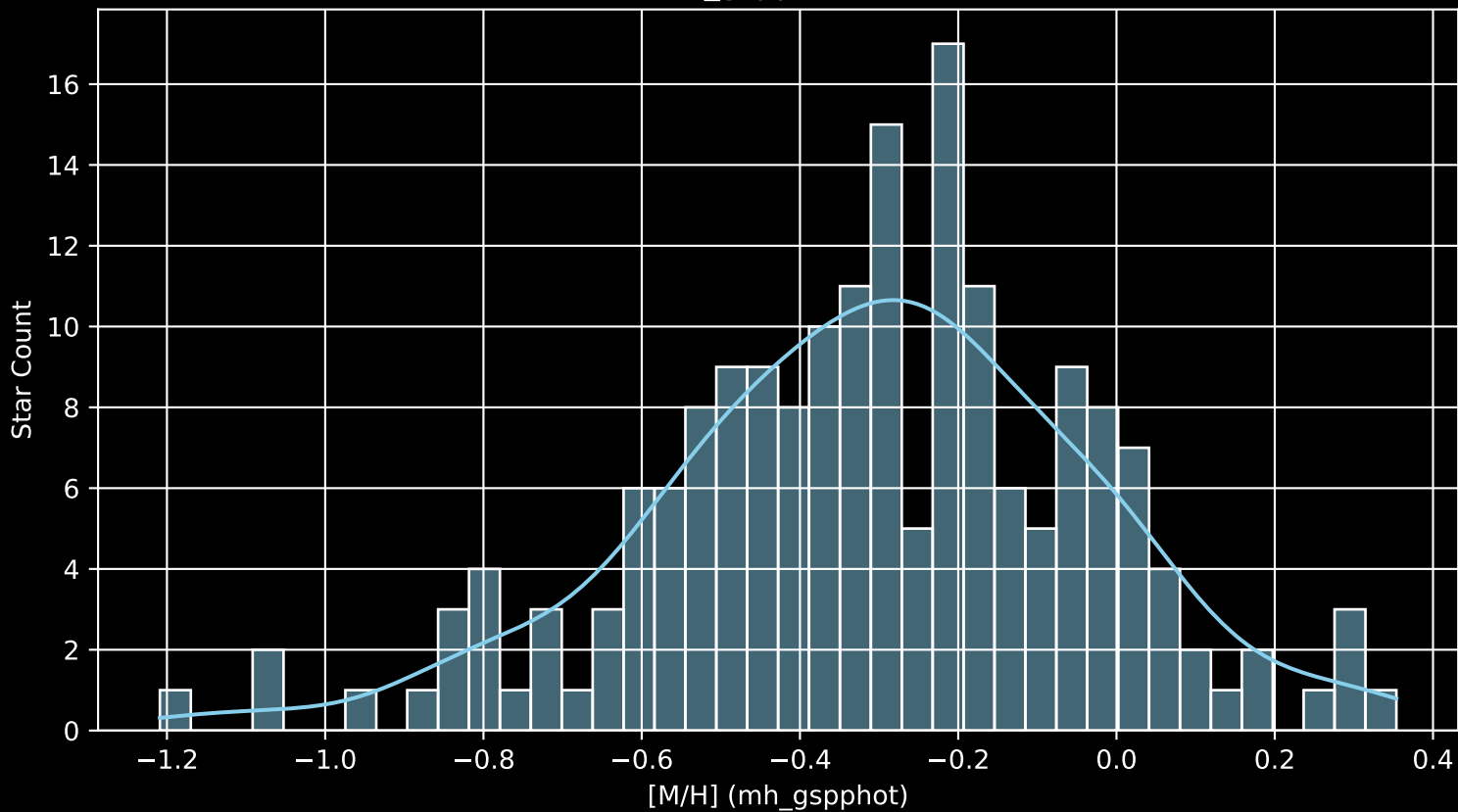
GALAH DR4 Field: [343] [M/H] (mh_gspphot) (n= 184)
