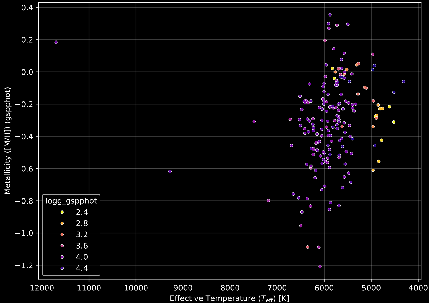
GALAH DR4 Field: [343] Stellar Population Parameters (n= 184)
