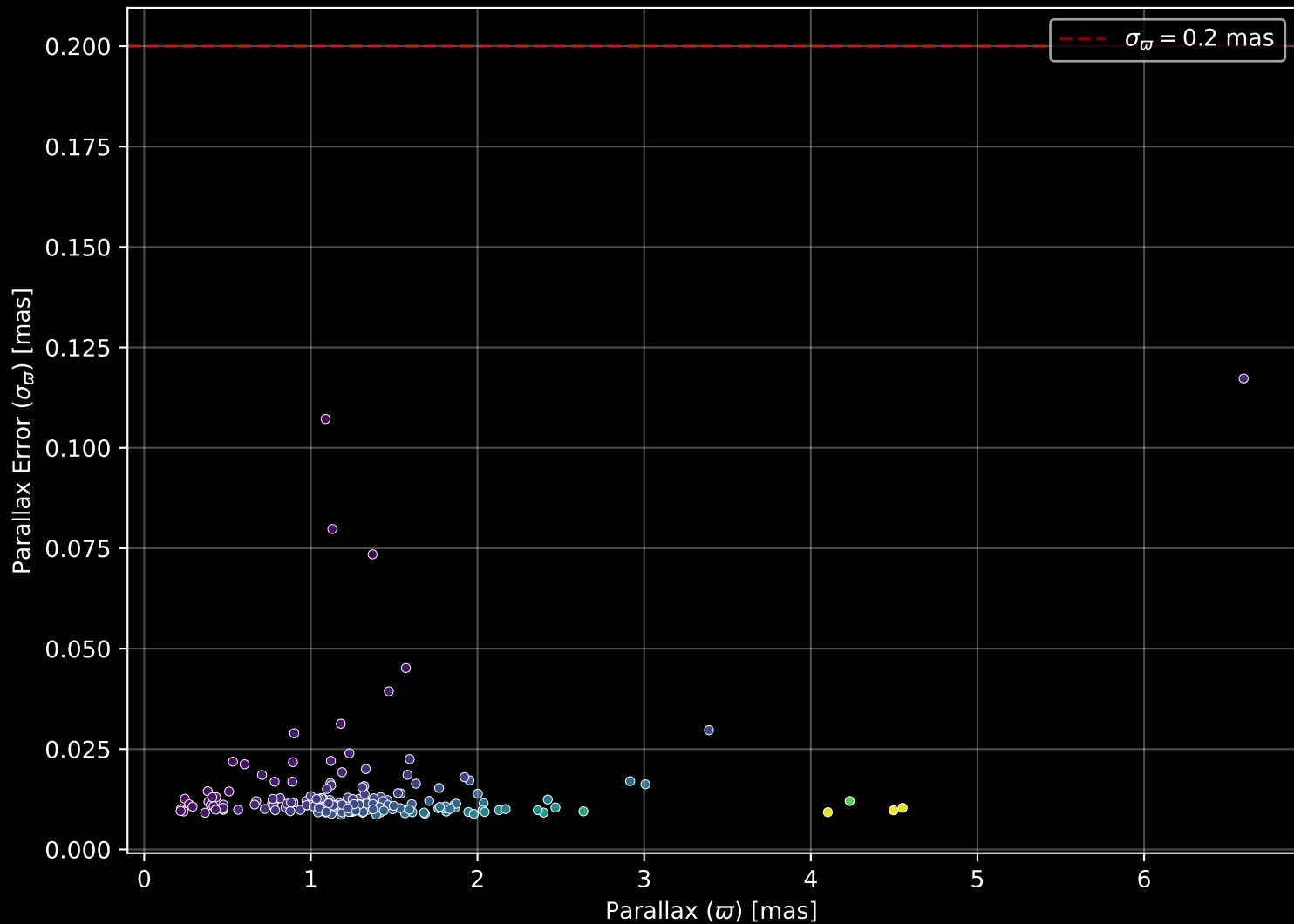
GALAH DR4 Field: [343] Parallax Quality (n= 184)
